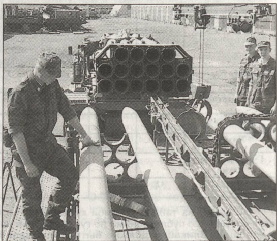
Артиллерийская установка
