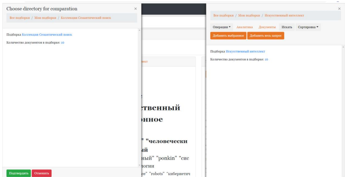
Рисунок 54 - Сравнение подборок
