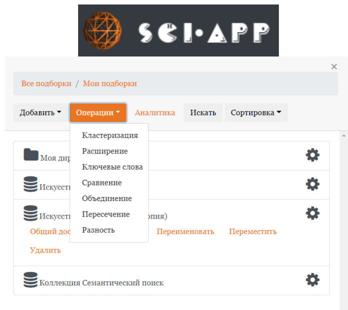
Рисунок 51 - Операции
