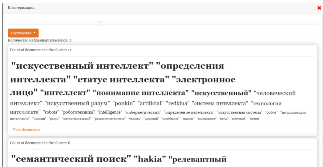
Рисунок 52 - Кластеризация
