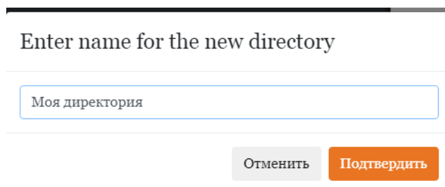
Рисунок 38 - Добавление директории
