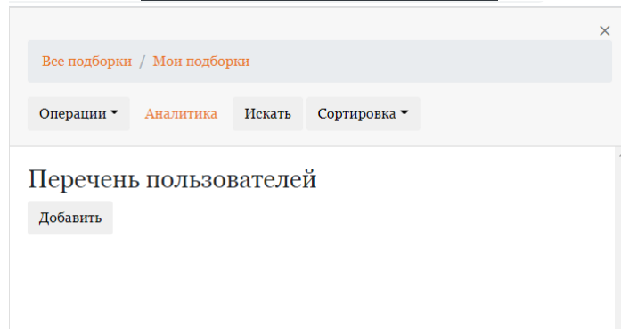
Рисунок 42 - Общий доступ
