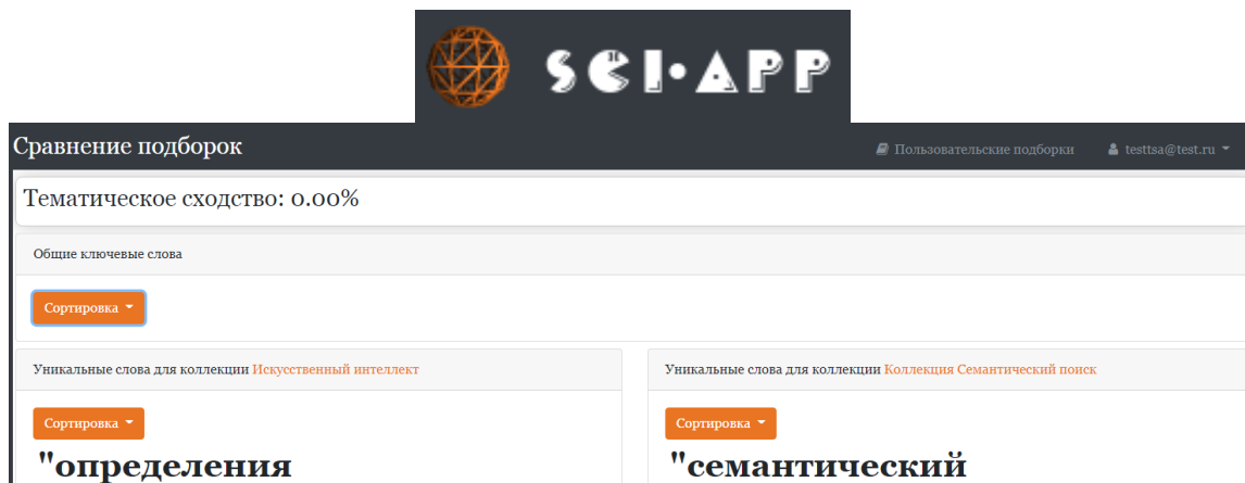
Рисунок 55 - Результат сравнения
