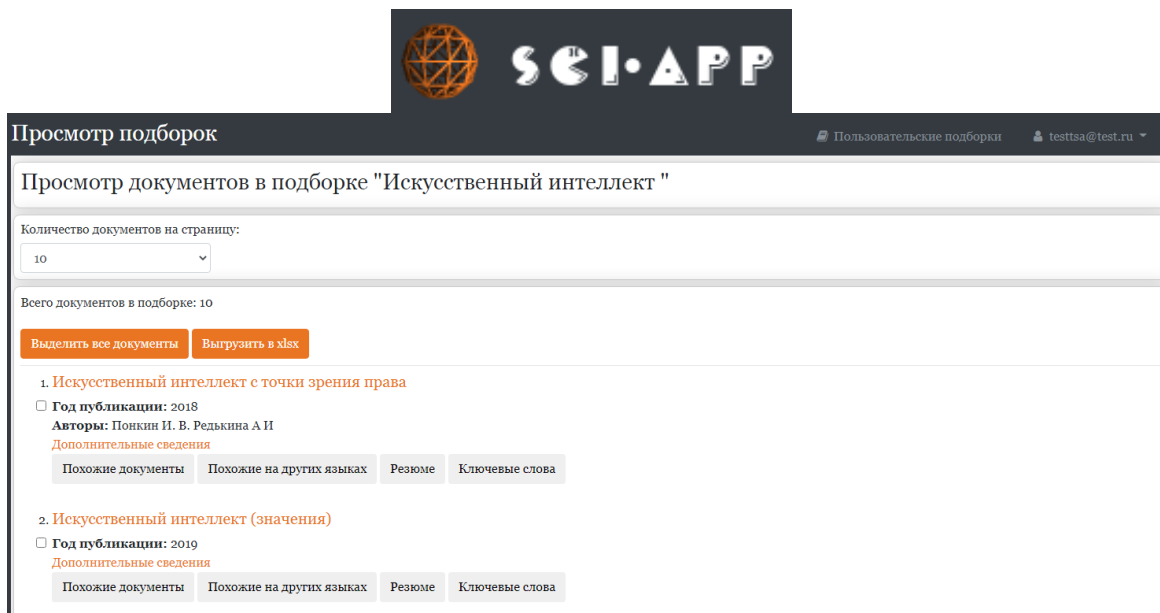
Рисунок 63 - Список документов
