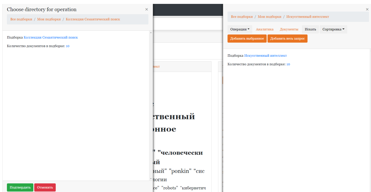
Рисунок 56 - Объединение
