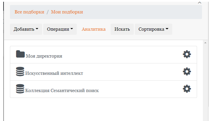
Рисунок 40 - Добавлены коллекции
