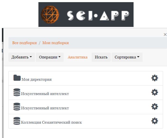
Рисунок 45 - Копия создана
