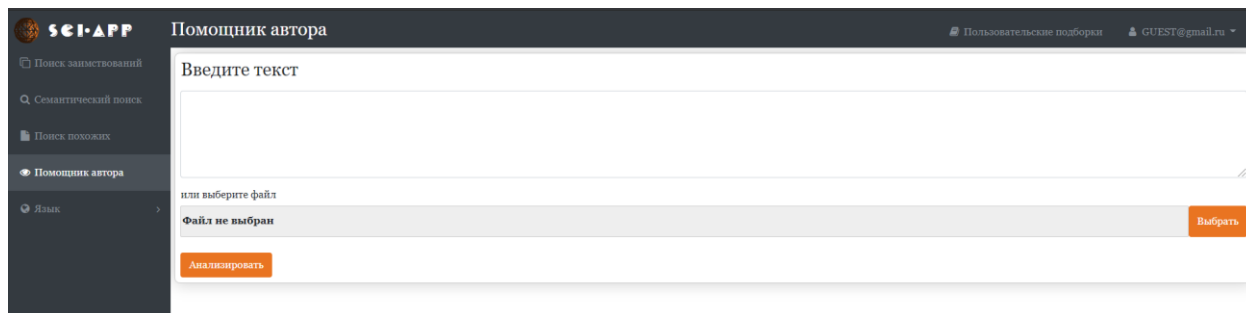
Рисунок 23 - Помощник автора
