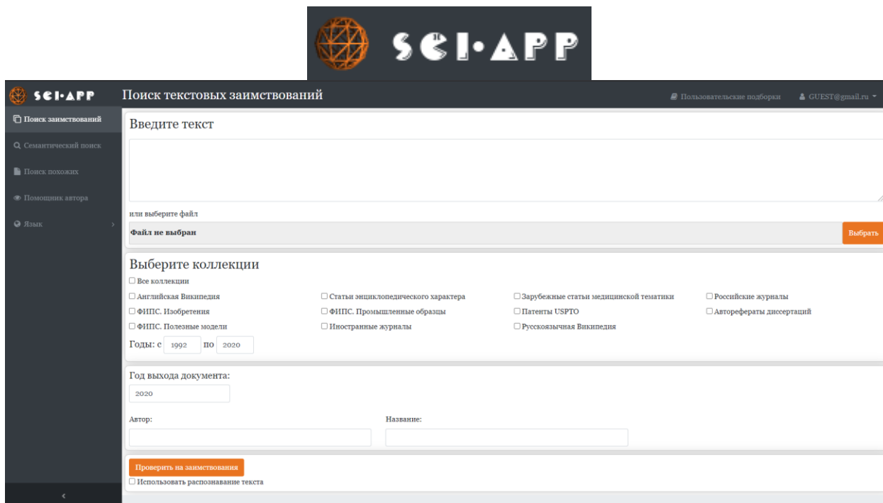
Рисунок 4 - Поиск заимствований
