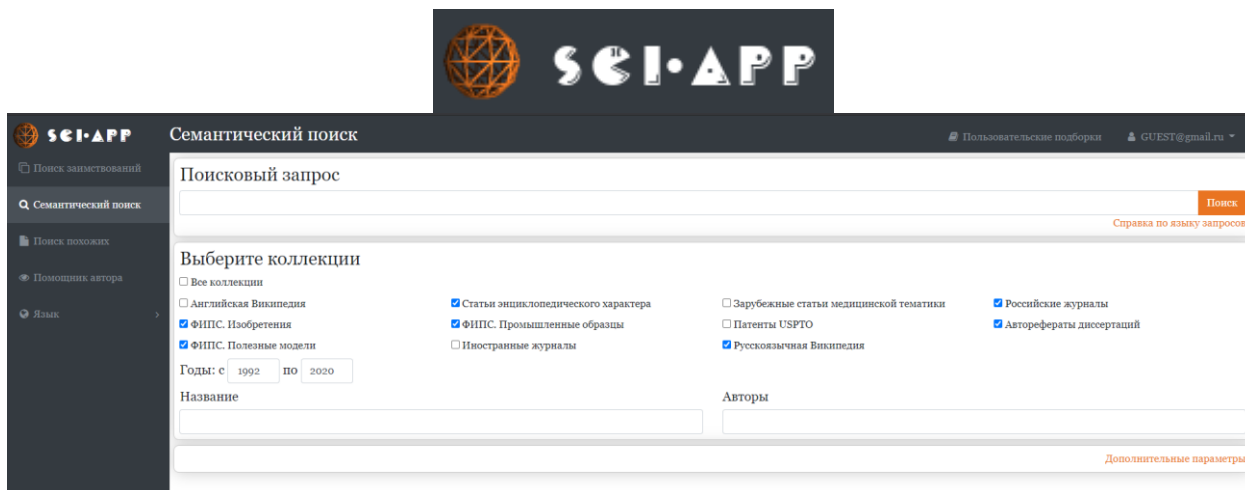
Рисунок 16 - Семантический поиск
