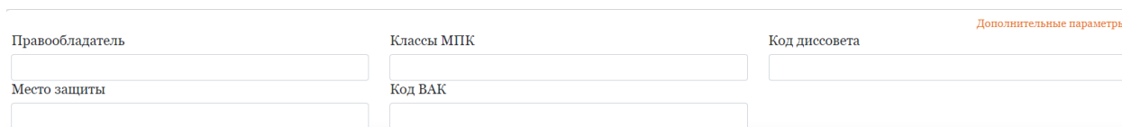
Рисунок 18 - Дополнительные параметры
