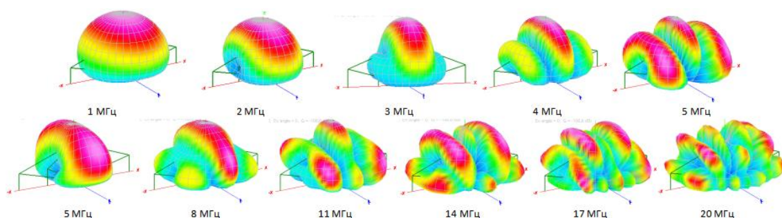
Рис. 1. Трехмерные диаграммы направленности большого ромба на частотах от 1 МГц до 5 МГц (сверху) и малого ромба на частотах от 5 до 20 МГц (снизу)
