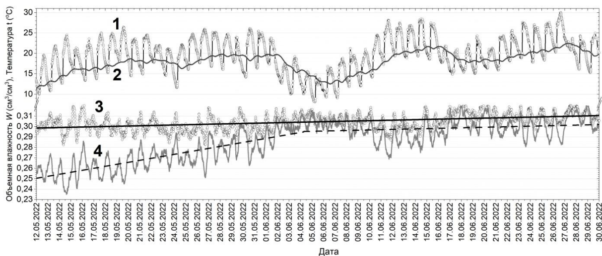
Рис. 1. Суточные вариации t_0(1) , t_{20}(2) , W_1(3) , W_2(4) в весенне-летний период
