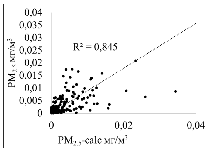
Рис. 1. Сравнение наземных данных (ось y ) и расчетных значений PM_{2.5}
