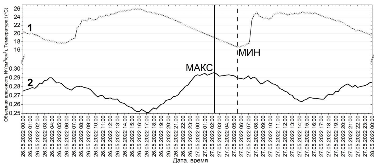
Рис. 2. Суточные колебания t_0(1) и W_2(2)
