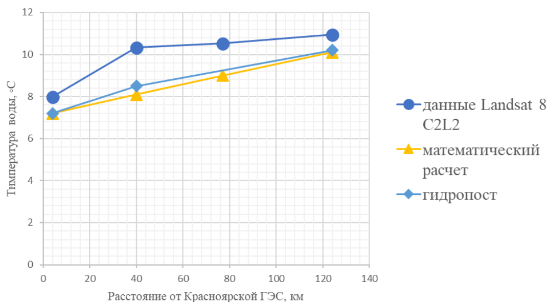
Рис. 2. Температура воды в нижнем бьефе Красноярской ГЭС
