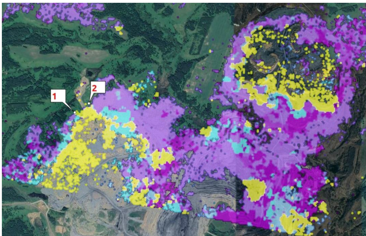
Рис. 3. Классы подвижности участков на подложке Google Satellite от стабильных (сиреневый) до нестабильных (желтый)
