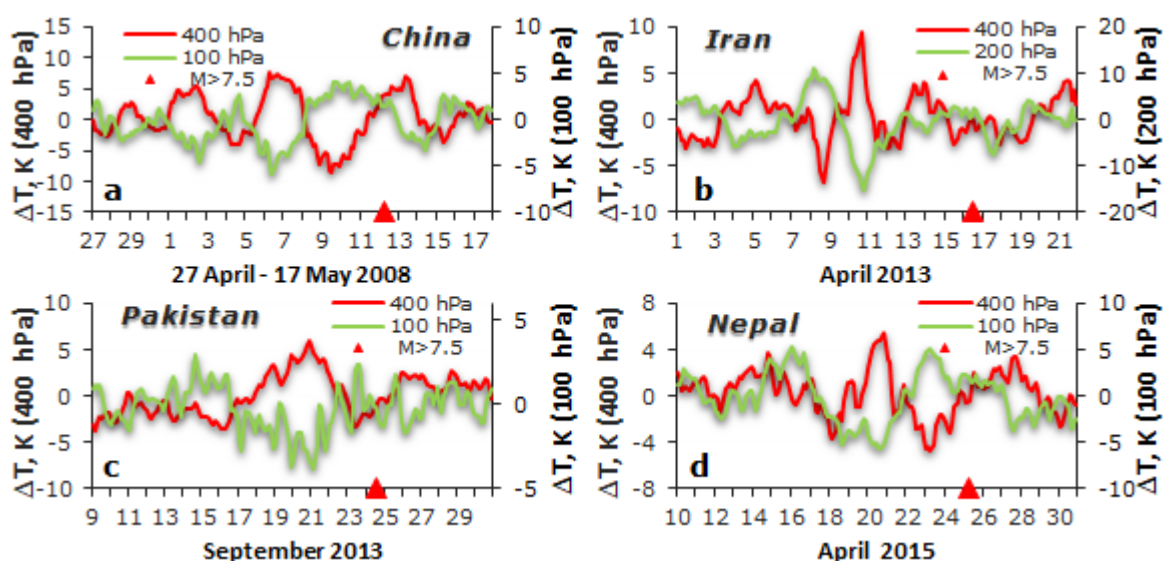
Рис. 1. Вариации приращений температуры \Delta T в верхней тропосфере (400 hPa) и области тропопаузы (200 и 100 hPa) в периоды сейсмической активности в Китае (a), Иране (b), Пакистане (c) и Непале (d). Маркерами отмечены моменты событий M > 7.5
