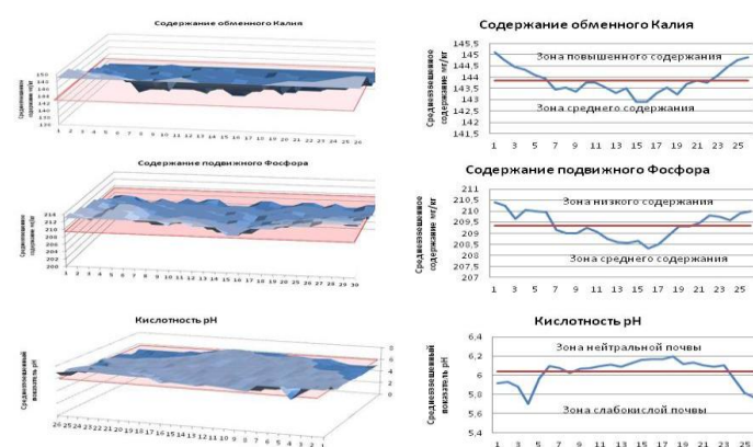
Рис. 1. Сегментация изображения средневзвешенных показателей обменного калия, подвижного фосфора и кислотности
