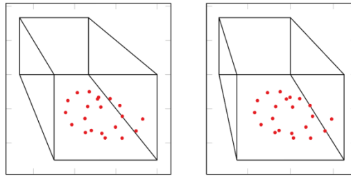
Рис. 4. Сечение x(t) = 0.7 в стереопроекции
