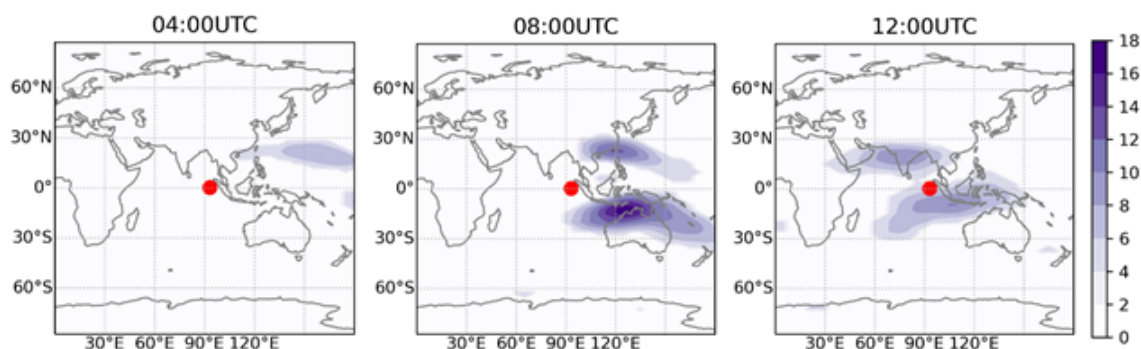
Рис. 1. Развитие во времени пространственного распределения аномалий ПЭС 05.04.2021 (за 6 дней до события M = 8.6 , эпицентр которого отмечен маркером)
