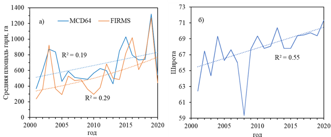
Рис. 1. Динамика средней площади гарей (а) и северное продвижение гарей (б). Тренд (б) построен без учета 2008 г.
