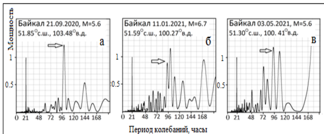
Рис. 2. Периодограммы Байкальских землетрясений 21 сентября 2020 г. (а), 11 января 2021 г. (б) и 3 марта 2021 г. (в)
