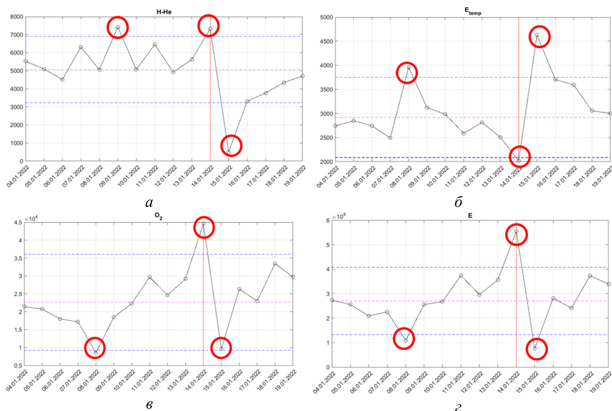
Рис. 2. Результаты обработки данных КА DMSP : а – концентрация ионов гелия и водорода; б – температура электронов; в – концентрация ионов кислорода; г – концентрация электронов
