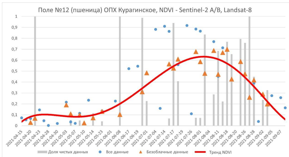
Рис. 2. Результат автоматизированного расчета NDVI для поля 12 ОПХ «Курагинское»
