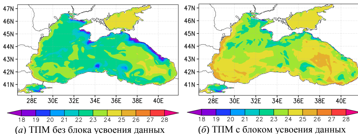
Рис. 1. Среднесуточные значения ТПМ на 1 июля 2019 г., рассчитанные по модели, °C
