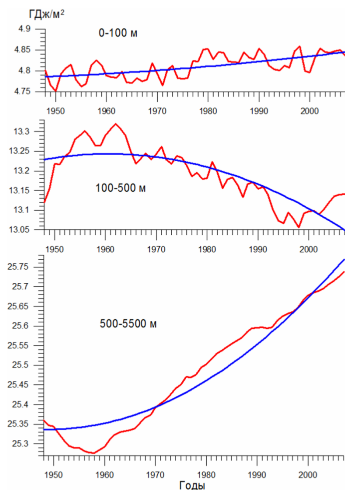
Рис. Изменчивость теплосодержания Мирового океана в период с 1948 по 2007 г.: в верхнем однородном слое (0–100 м), в слое главного термоклина (100–500 м) и в глубинном слое (500–5 500 м)
