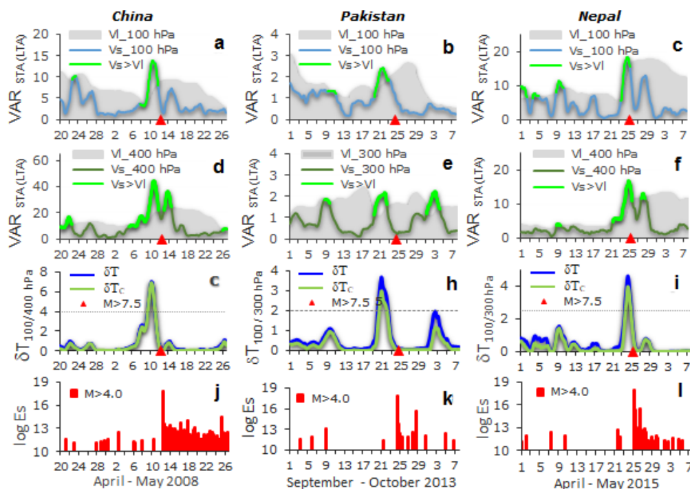
Рис. 2. Временные ряды скользящих дисперсий VAR_{STA} и VAR_{LTA} на уровнях 100 hPa ( a, b, c ) и 300–400 hPa ( d, e, f ); соответствующие вариации \delta T и \delta T_C ( g, h, i ) над эпицентрами землетрясений M > 7.5 ; распределение логарифма сейсмической энергии ( \log Es ) ( j, k, l ) в рассматриваемые периоды в Китае (20 апреля – 26 мая 2008 г.), Пакистане (1 сентября – 7 октября 2013 г.) и Непале (1 апреля – 7 мая 2015 г.)
