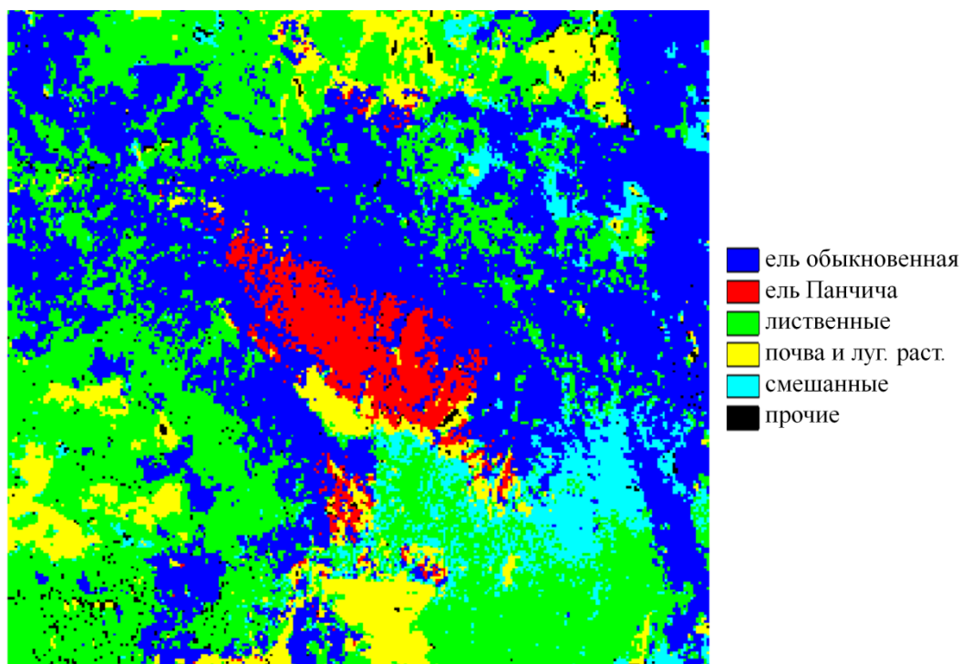
Рис. 2. Классификация основных типов объектов тестовой территории по данным Sentinel-2 . Насаждения ели Панчича выделены красным цветом
