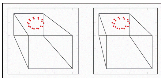
Рис. 3. Сечение x(t) = 0.2 в стереопроекции
