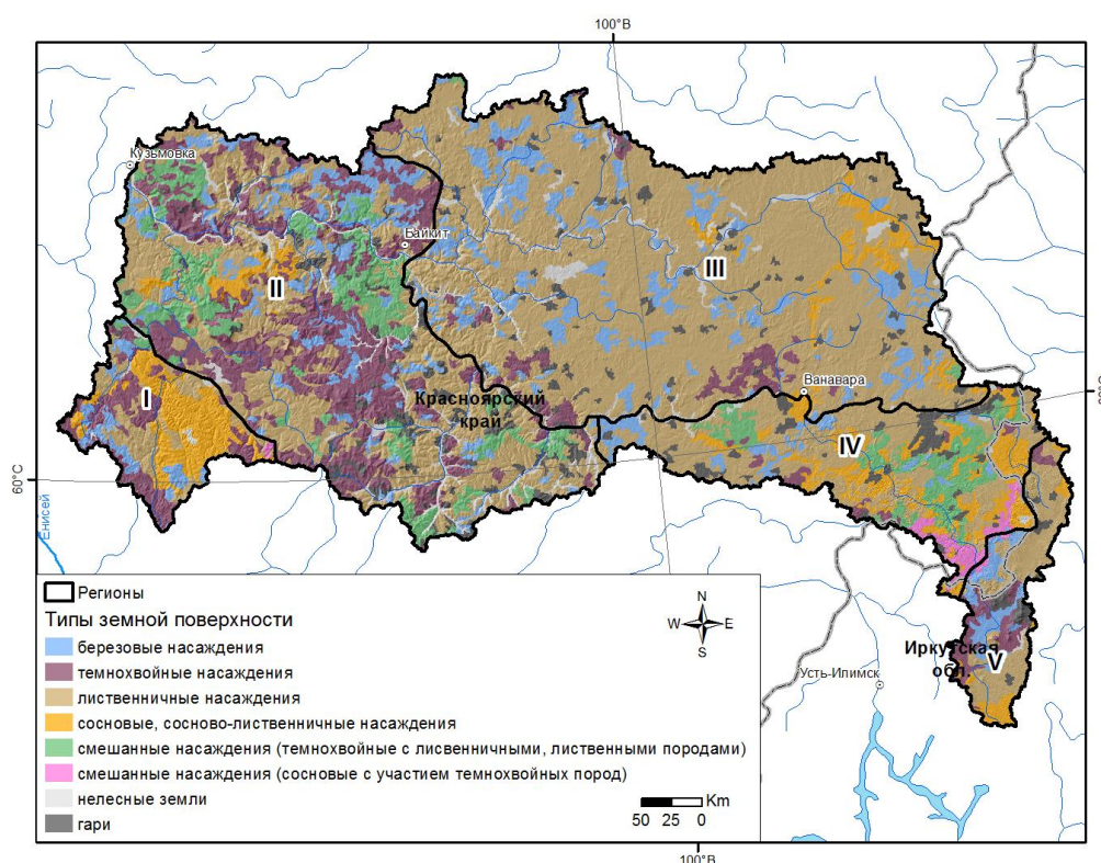
Рис. Распределение типов земной поверхности и регионов в бассейне реки Подкаменная Тунгуска
