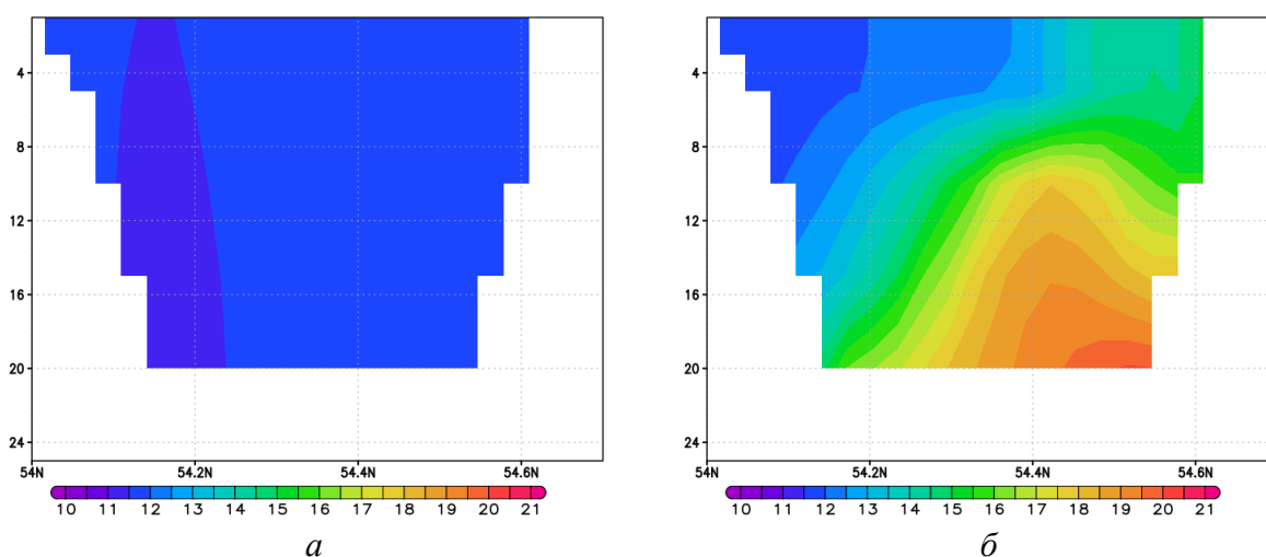
Рис. Значения солёности (е.п.с.) в проливе Фемарн-Бельт на долготе 11,4^\circ : а – на 28.12.2014, результат расчета с использованием ньютоновской релаксации к данным наблюдений; б – на 28.12.2014, результат расчета с использованием вариационной ассимиляции
