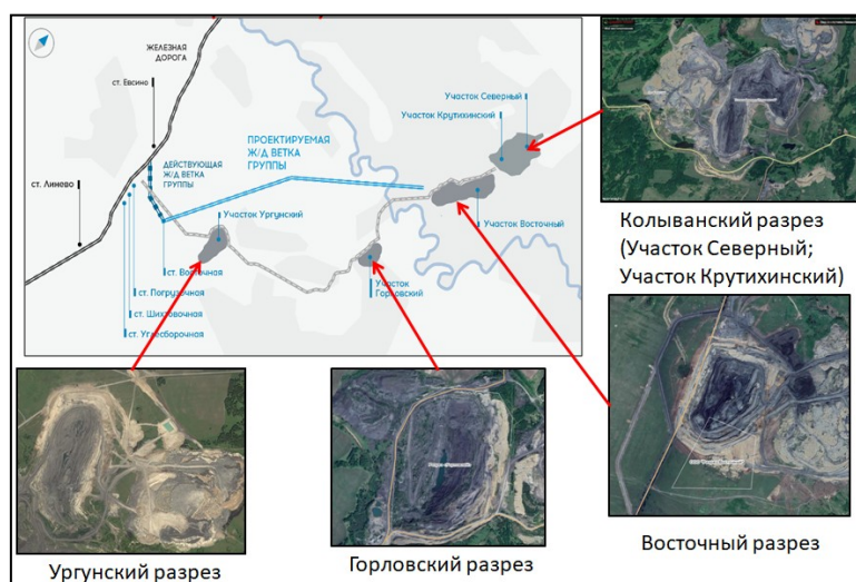
Рис. 1. Схема Горловского угольного бассейна
