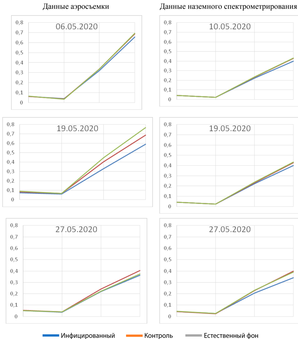
Рис. Динамика КСЯ на экспериментальных участках с посевами озимой пшеницы (Каждому вертикальному делению соответствуют диапазоны волн: 550, 660, 735 и 790 нм)
