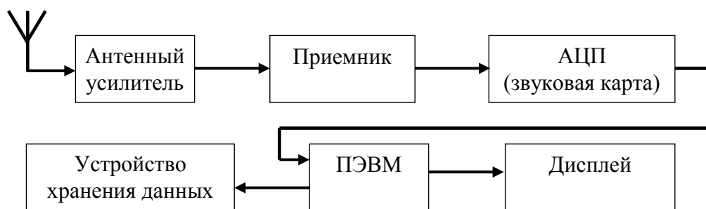
Рис. Структурная схема экспериментального АПК
