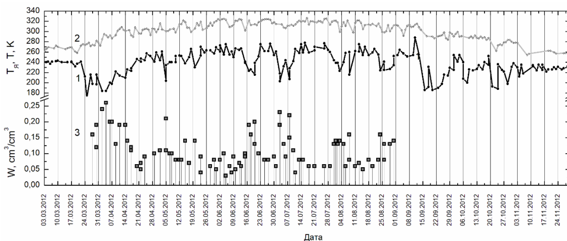
Рис. 2. Сезонная динамика радиояростной (1), физической (2) температур подстилающей поверхности, объемной влажности W (3) ячейки № 4010460 ISEA 4H9
