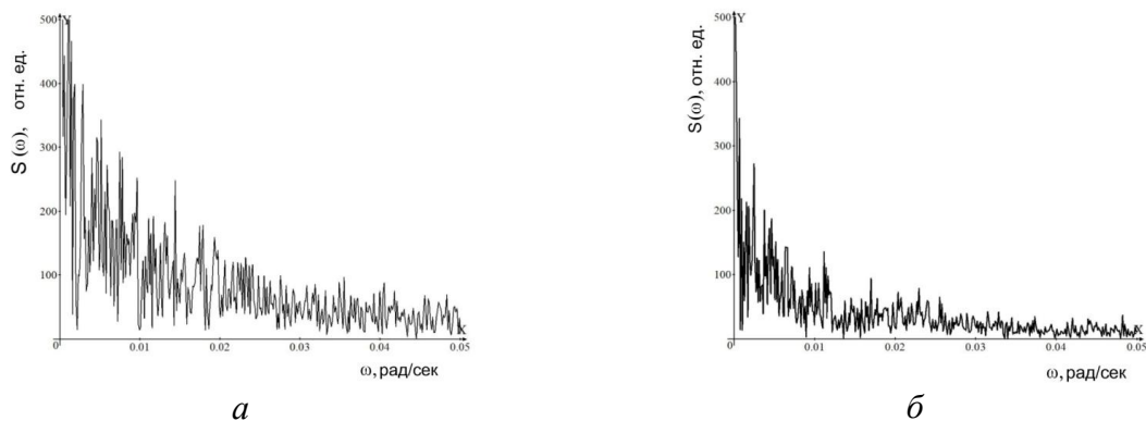
Рис. 2. Спектры Фурье S(\omega) : а – ТИ № 1, НС Galileo 2; б – ТИ № 2 НС Galileo 11
