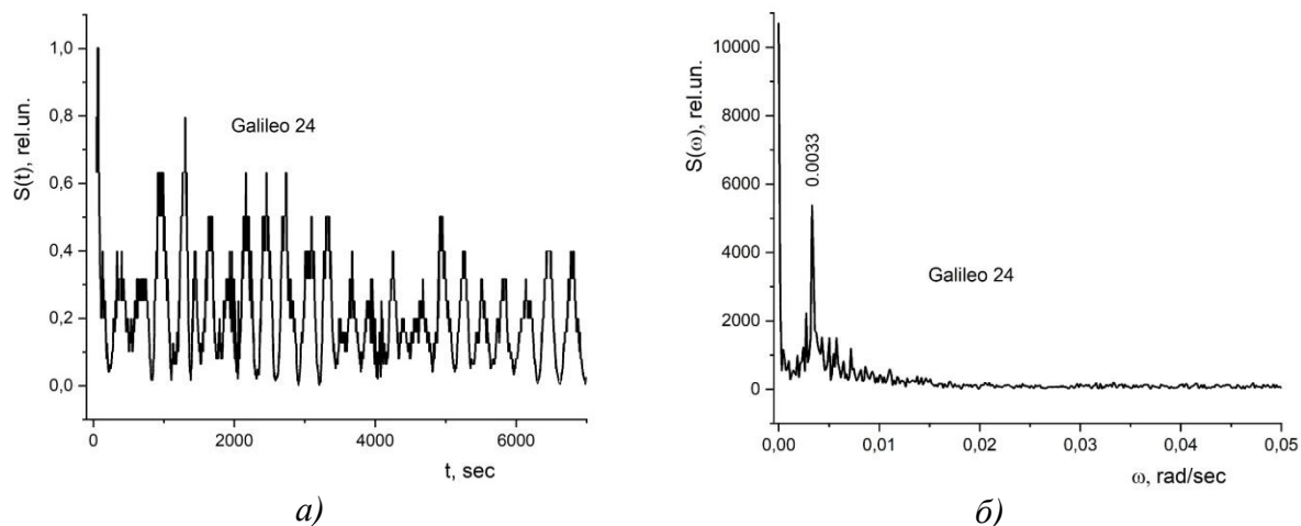
Рис. 3. Зависимости: a - S(t) , b - S(\omega) ; НС Galileo – 24, толщина льда 76 см
