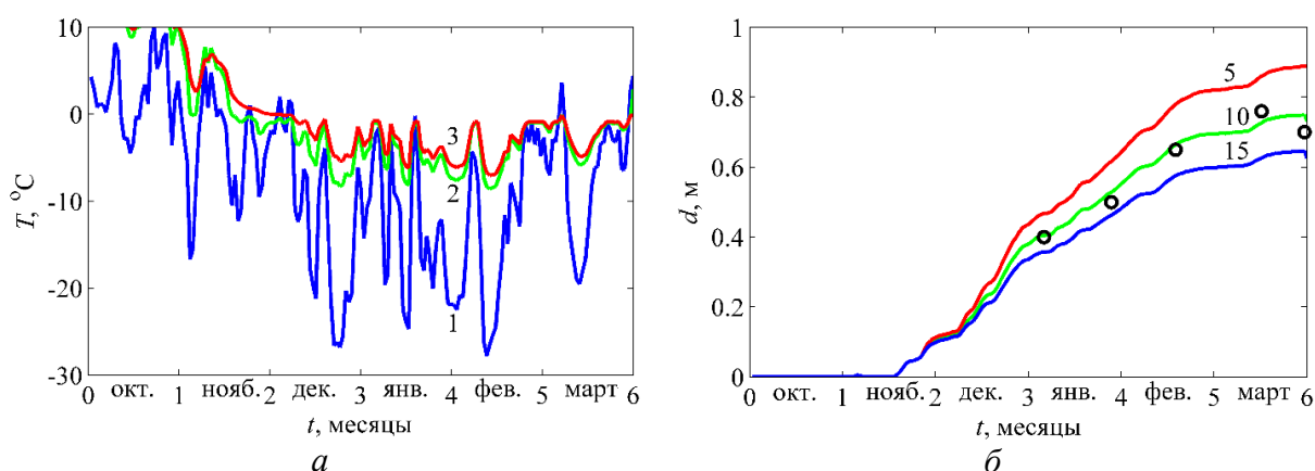
Рис. 1. Временные зависимости температуры ( а ) и толщины слоя льда ( б )
