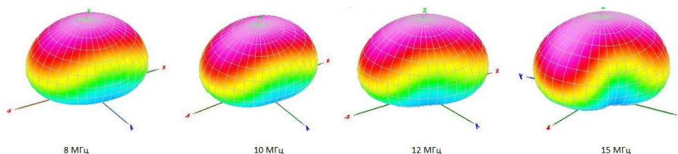
Рис. 4. Трехмерные диаграммы направленности антенны типа скрещенный диполь на частотах от 8 МГц до 15 МГц
