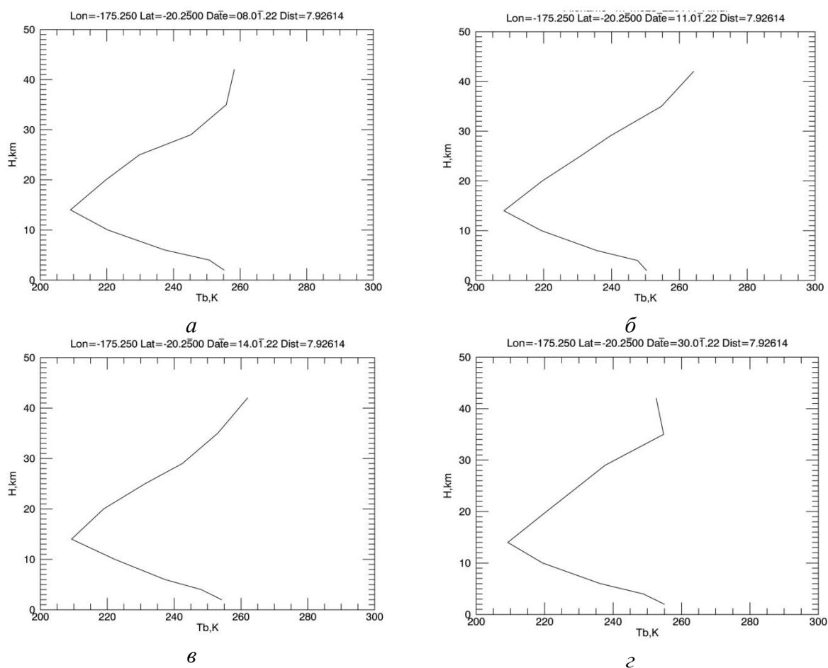
Рис. 1. Профили радиоярких температур 08.01.22 ( a ), 11.01.22 ( б ), 14.01.22 ( в ), 30.01.22 ( г )
