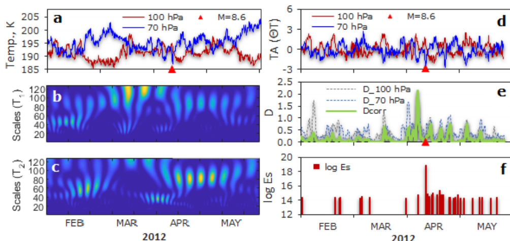
Рис. 2. Временные ряды температуры T_1 и T_2 на уровнях 100 и 70 гПа ( a ), спектры коэффициентов вейвлет-преобразования ( b , c ), аномалии температуры \Delta T ( d ), параметр D_{CORR} ( e ), логарифм сейсмической энергии \log(Es) ( f ) в период с февраля по май 2012 г.
