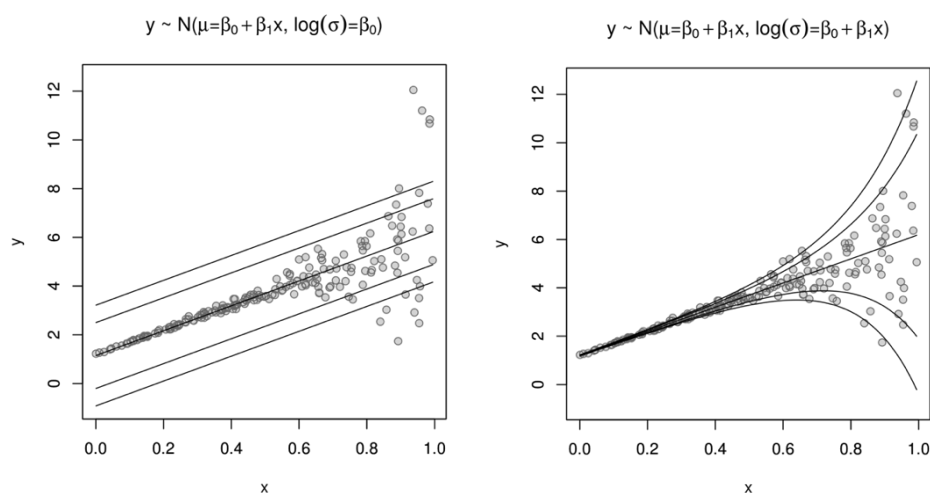
Рис. 1. Пример смоделированных данных, показаны расчетные 2.5 %, 10 %, 50 %, 90 % и 97.5 % квантилей гомоскедастической нормальной модели слева и гетероскедастической нормальной модели справа
