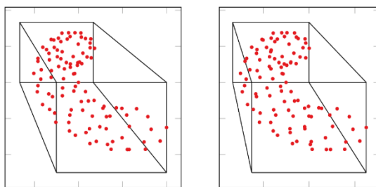
Рис. 2. Множество S_1 в стереопроекции
