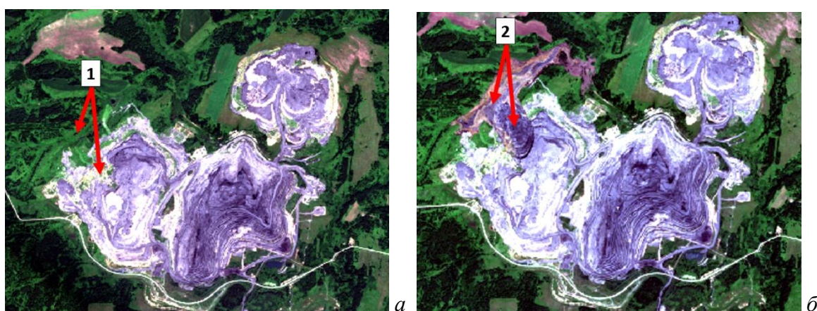
Рис. 2. Изображения исследуемой области (Sentinel-2, фильтр RGB): а – до события (16.07.2020); б – после события (19.07.2020)
