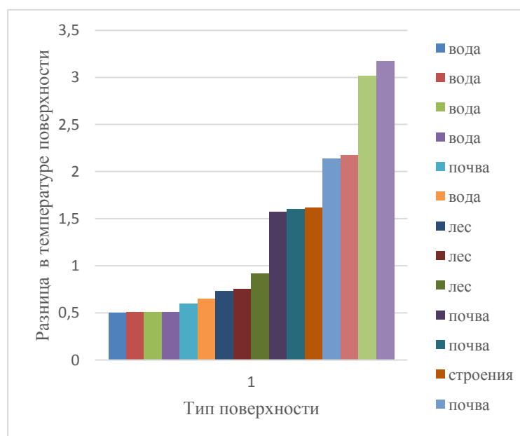
Рис. 2. Соотношение разницы температур к типу подстилающей поверхности
