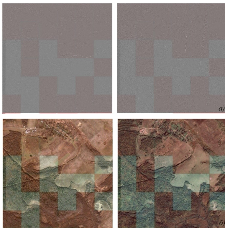
Рис. Фрагменты вейвлет-образов и снимков QuikBird , WorldView
