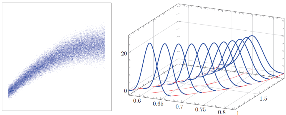
Рис. 2. Модель исходных данных (слева) и график аппроксимации функций плотности вероятности максимальных значений
