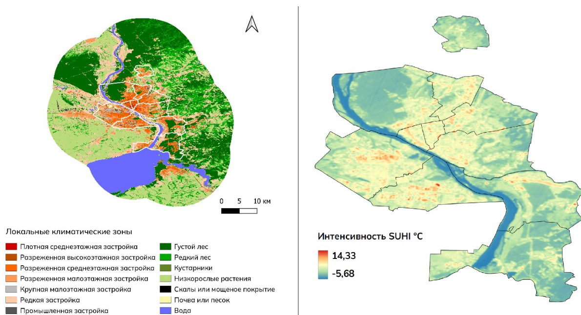
Рис. 1. Карта LCZ Новосибирска и его окрестностей (слева), и значения интенсивности SUHI для всех LCZ внутри города за 12.07.18 (справа)
