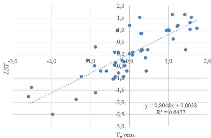
Рис. Регрессионная зависимость стандартизованных значений LST и T_{п\text{ }max}
