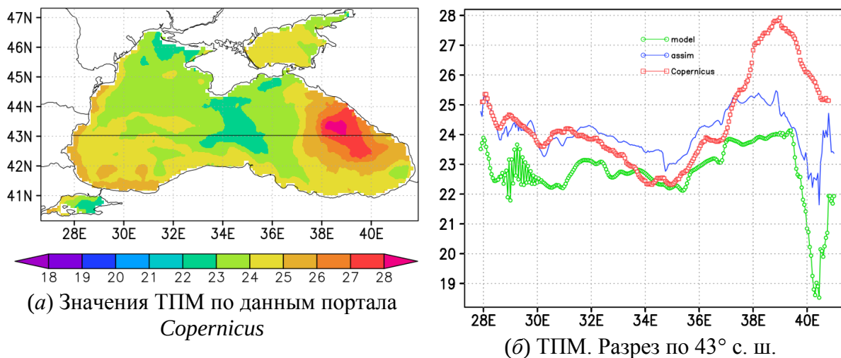
Рис. 2. Среднесуточные значения ТПМ на 1 июля 2019 года, °C
