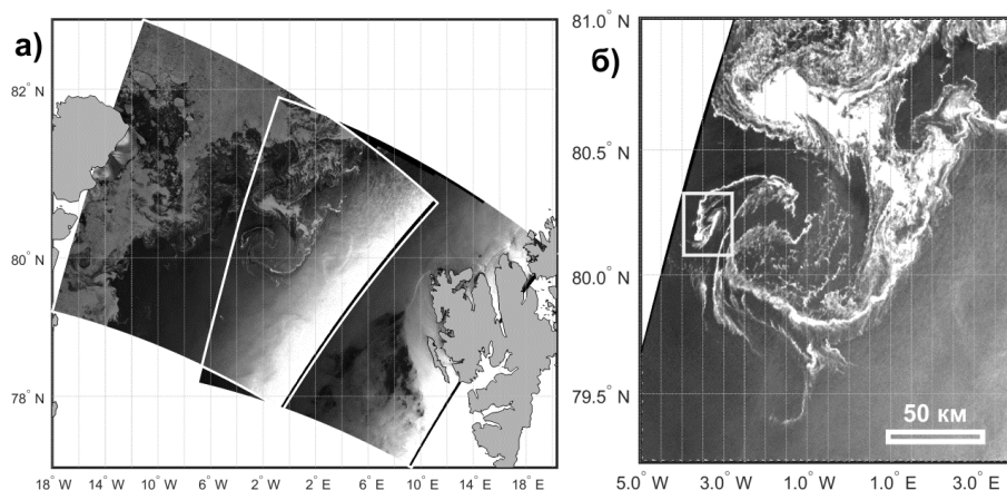
Рис. 1. а ) Положение двух квазисинхронных РЛИ Sentinel-1 A/B за 17 сентября 2017 г. в районе пролива Фрама; б ) Фрагмент РЛИ Sentinel-1A за ту же дату (07:12 UTC) с отчетливым проявлением антициклонического вихря в прикромочной ледовой зоне
