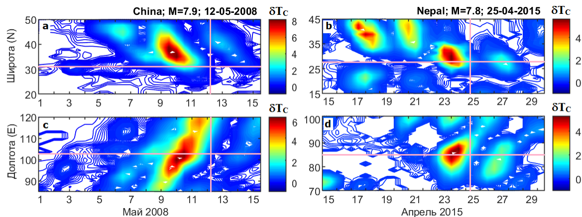
Рис. 3. Распределения параметра \delta T_C по широте ( a, b ) и долготе ( c, d ) в Китае (с 1 по 15 мая 2008 г.) и Непале (с 15 по 30 апреля 2015 г.) Вертикальные и горизонтальные линии указывают моменты землетрясений и координаты их эпицентров
