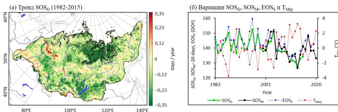
Рис. 1. а – карта тренда SOS_G на территории Сибири за 1982–2015 гг. Точками отмечены области с p < 0,05 . Черной линией выделена область ROI; б – межгодовые вариации SOS_G , SOS_M , EOS_S и T_{May} для ROI
