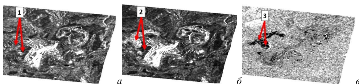
Рис. 1. Изображения исследуемой области (Sentinel-1 GRD) со значениями показателей обратного рассеяния: а – до события (16.07.2020); б – после события (19.07.2020); в – результирующее изображения с некогерентным изменением
