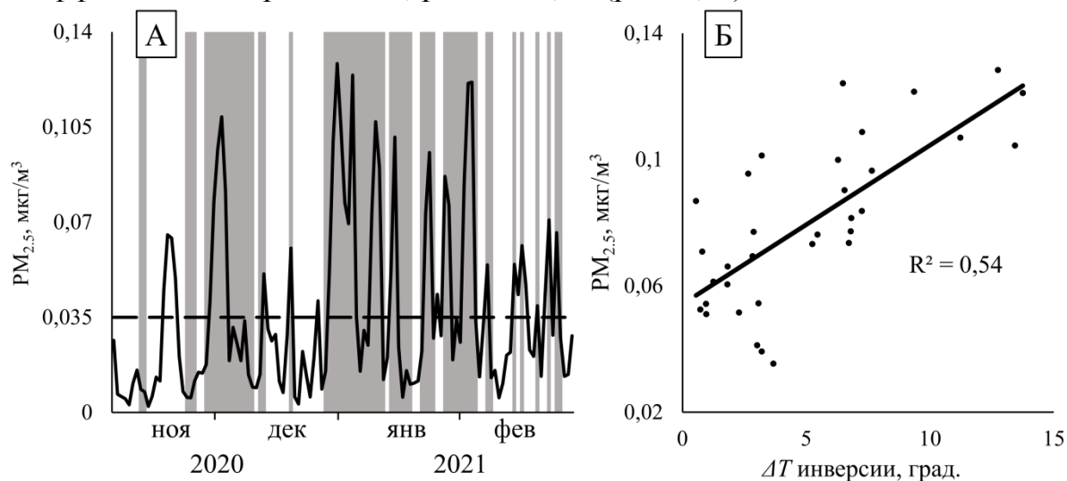
Рис. 1. Взаимосвязь среднесуточных концентраций PM_{2.5} и температурных инверсий в Красноярске в холодный сезон 2020–2021 г.
