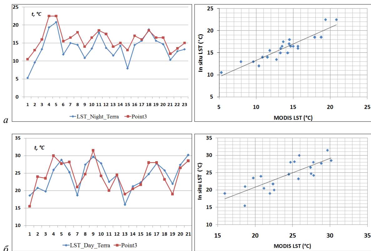
Рис. Примеры графиков динамики ночных (а) и дневных (б) температур и диаграмм рассеяния, полученных на основе наземных и спутниковых измерений (MODIS/Terra) в точке 3 за период 09.06.2021–20.09.2021
