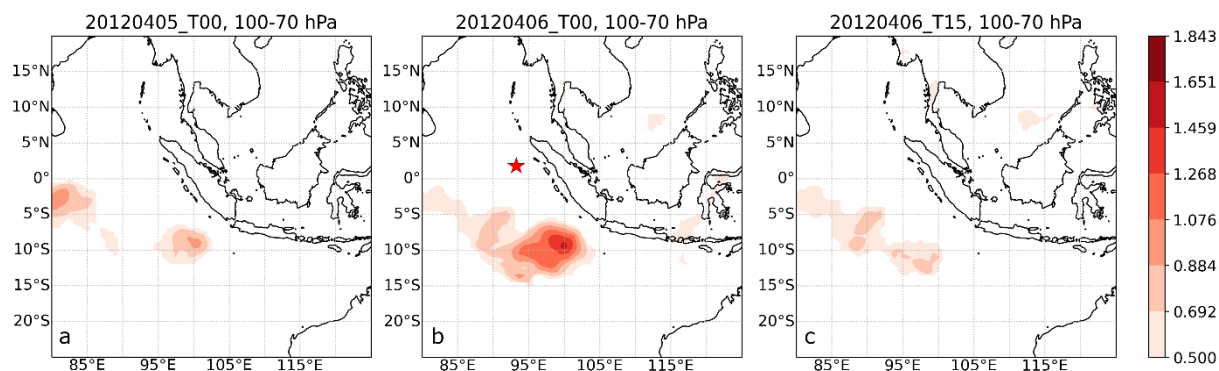
Рис. 3. Эволюция пространственного распределения температурной аномалии 05.04.2012 (00:00 UTC) ( a ), 06.04.2012 (00:00 UTC) ( b ) и 06.04.2012 (15:00 UTC) ( c ). Эпицентр сейсмического события (93.063 °E; 2.327 °N) отмечен красным маркером
