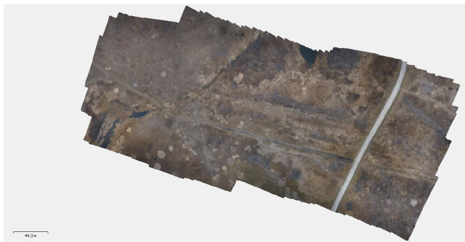
Рис. 3. Полученный ортофотоплан в Agisoft Metashape
