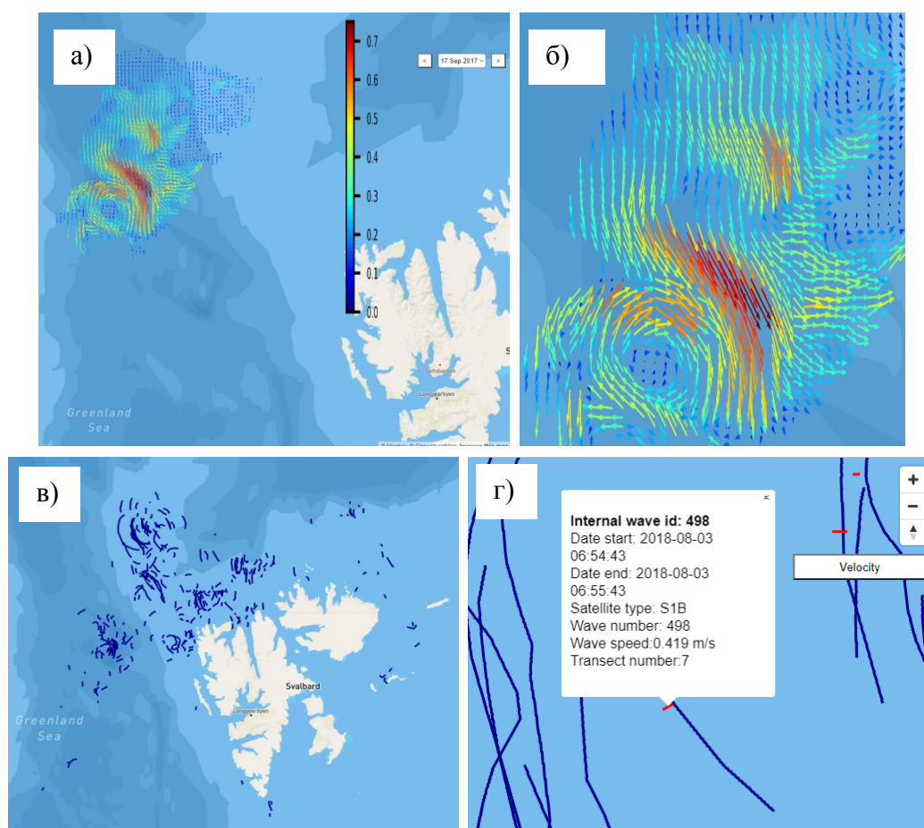
Рис. 2. Примеры спутниковых продуктов на сайте http://polar-space.ru , полученных на основе обработки квазисинхронных РЛИ Sentinel-1 A/B для пролива Фрама. Вверху ( а , б ) – скорость дрейфа льда внутри ПЛЗ с антициклоническим вихрем, внизу – лидирующие гребни внутренних волн ( в ) и значения их фазовой скорости ( г )
