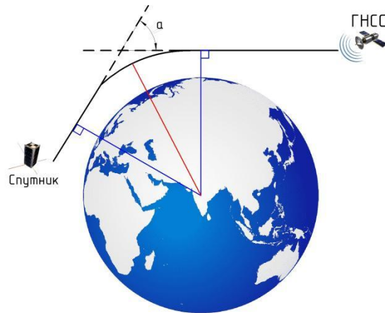
Рис. Геометрическое определение затмения сигналами спутников ГНСС
