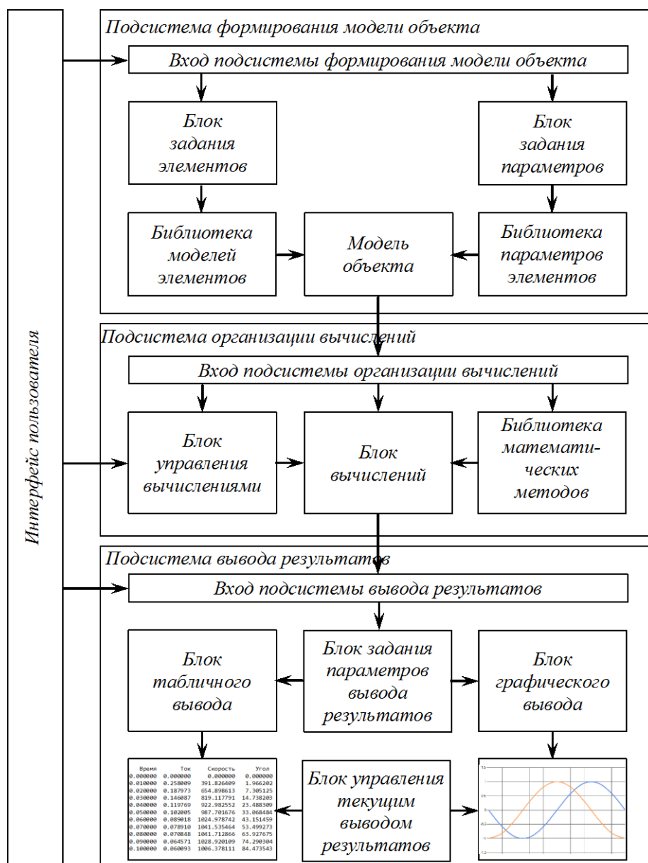
Рис. Структурная схема системы моделирования
