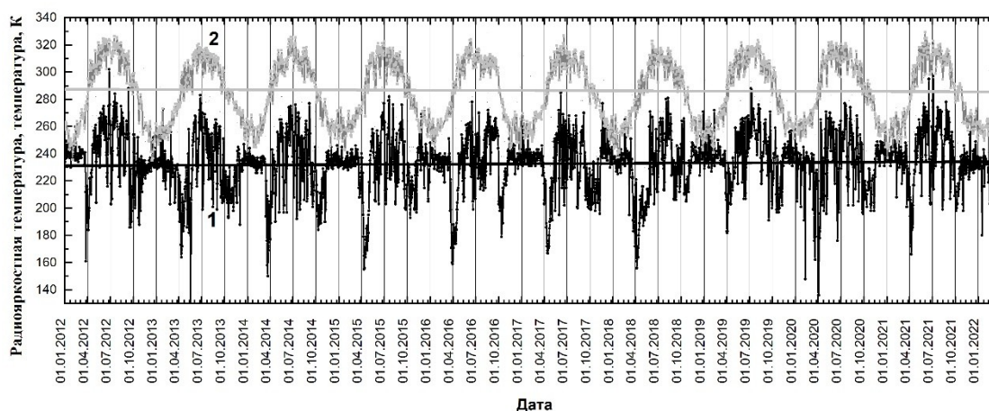
Рис. 1. Многолетняя динамика радиояростной (1) и физической (2) температур подстилающей поверхности ячейки № 4010460 ISEA 4H9
