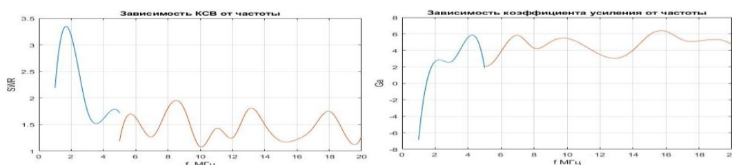
Рис. 2. КСВ стоячей волны (слева) и коэффициент усиления G_a в Dbi (справа) по диапазону частот. Синяя – большой ромб РА, красная – малый
