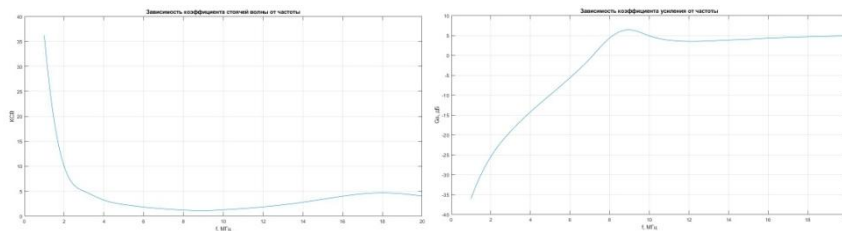
Рис. 3. КСВ стоячей волны (слева) и коэффициент усиления G_a в Dbi (справа) по диапазону частот. Синяя – большой ромб РА, красная – малый
