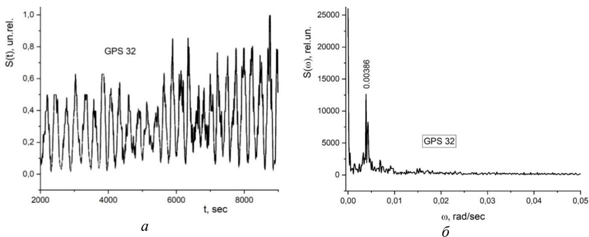
Рис. 2. Зависимости: a - S(t) ; b - S(\omega) ; НС GPS – 32, толщина льда 42 см
