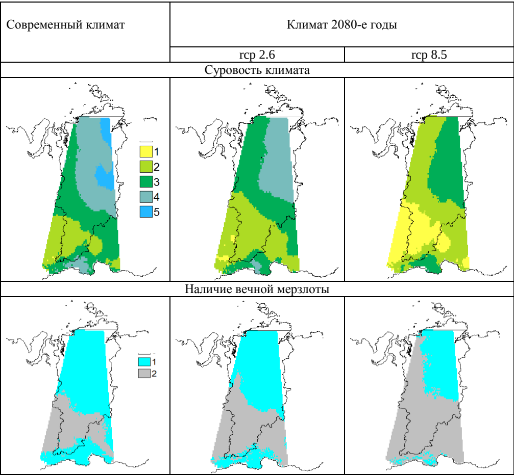
Рис. 2. Степень суровости климата (верхний ряд): 1 – относительно благоприятный; 2 – умеренный; 3 – неблагоприятный; 4 – суровый; 5 – экстремальный. Присутствие вечной мерзлоты (нижний ряд): 1 – зона вечной мерзлоты; 2 – территория, свободная от вечной мерзлоты
