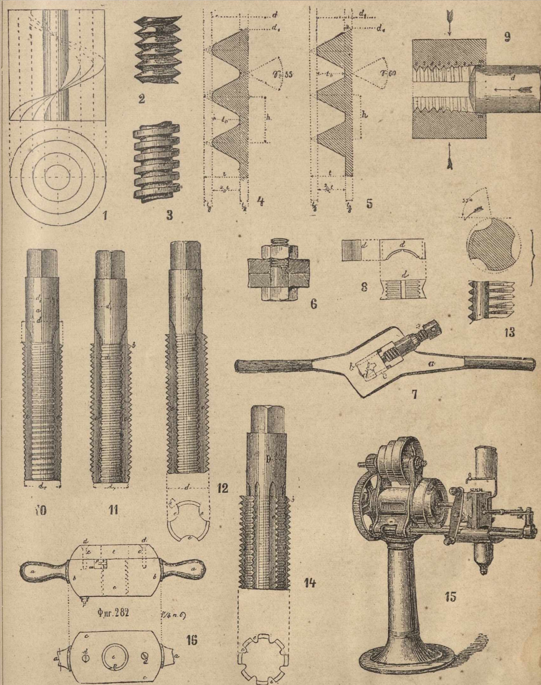
1) Витовая линия. Нарѣзки: 2) треугольная, 3) квадратная. 4) Витворта. 5) Селлерса. 6) Болтъ. 7) Клунка. 8) Плашки. 9) Дѣйствіе плашекъ Селлерса. 10 и 11) Мѣтки коническіе. 12) Цилиндрическій. 13) Селлерса. 14) Нормальный. 15) Болторѣзная машина. 16) Винтельна.
