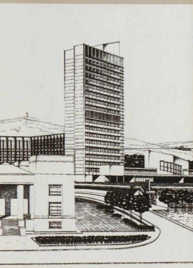
Здание Управления Енисейского речного пароходства (ЕнУРП) в Красноярске. Соавтор: Л.Л. Францева. 1969-1985
