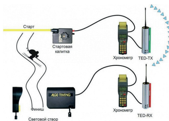
Рис. 2. Беспроводная система хронометража
